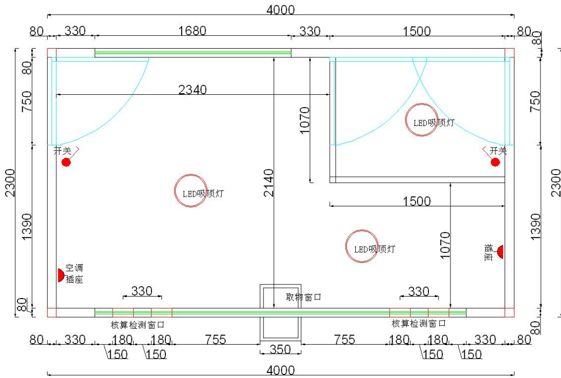
平面图
